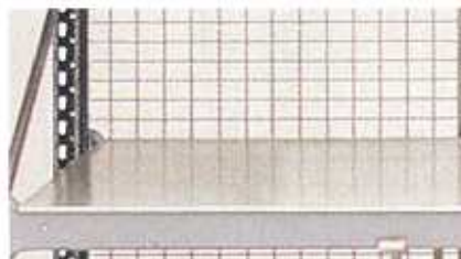
Täckta bärplan gör det möjligt att lagra ej pallat smågods på bärplanet.
